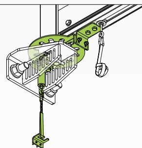
Sposób montażu Typical layout
