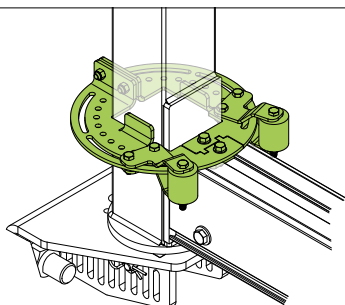
Sposób montażu Typical layout
